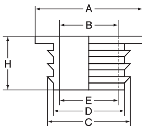
アダプター寸法表
