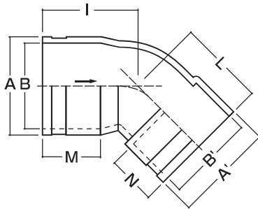
45°エルボタイプ寸法表
