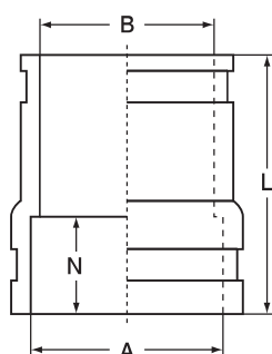
片側銅管タイプ寸法表
