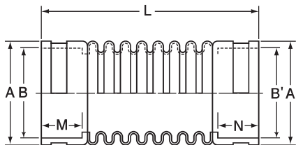
Mタイプ(ジャバラ)寸法表
