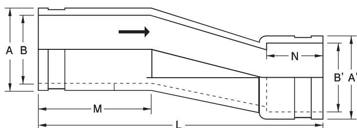
偏芯タイプ寸法表
