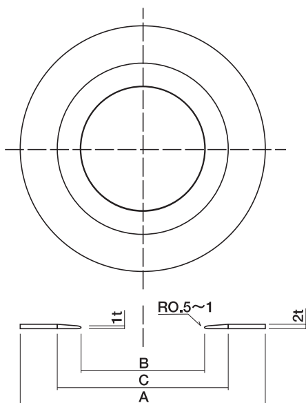
SGゴムプレート寸法表
