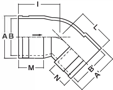
45°エルボタイプ寸法表
