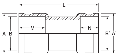
ソケットタイプ寸法表
