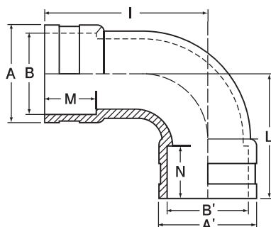
90°エルボタイプ寸法表
